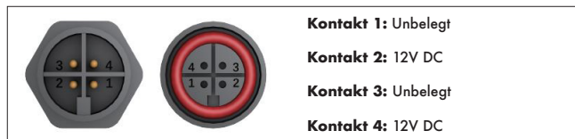
Abb.4: Kontaktbelegung des Motor-Steckverbinders
