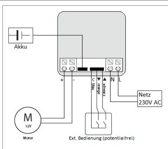
Abb.2: Anschlusskizze Tastor Lux Plus 12V
